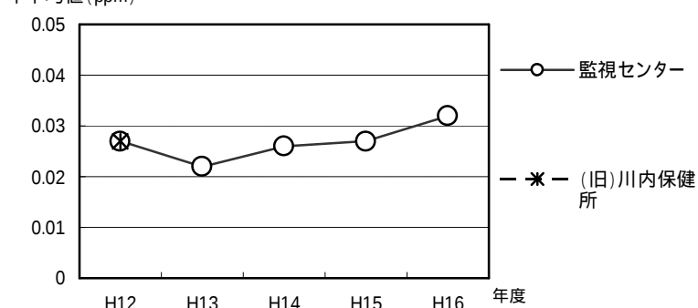
年平均値 (ppm) 図表 3-6 光化学オキシダント濃度の推移
