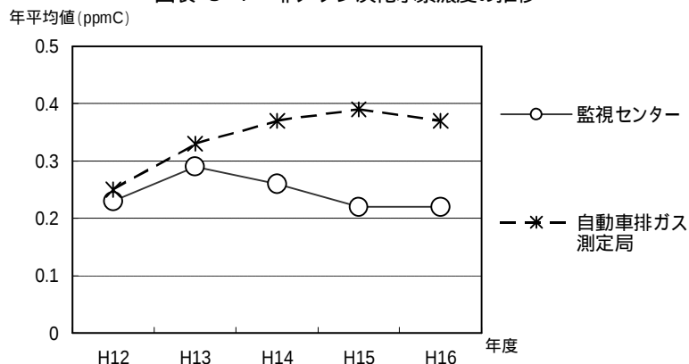
図表 3-7 非メタン炭化水素濃度の推移
