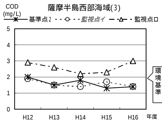
図表 3 -1 3 海域の水質の経年変化
