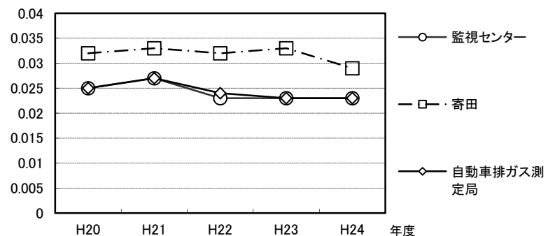
年平均值(ppm) 図表 3-4 浮遊粒子状物質濃度の推移
