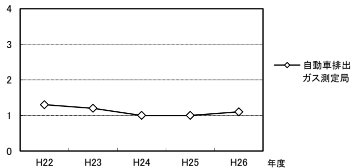
年平均値 ( \mu\text{g}/\text{m}^3 ) 図表 3-9 ベンゼン濃度の推移
