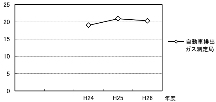
年平均値 ( \mu\text{g}/\text{m}^3 ) 図表 3-8 微小粒子状物質濃度の推移
