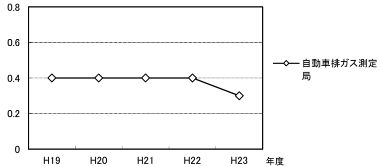
年平均值 (ppm) 図表 3-5 一酸化炭素濃度の推移
