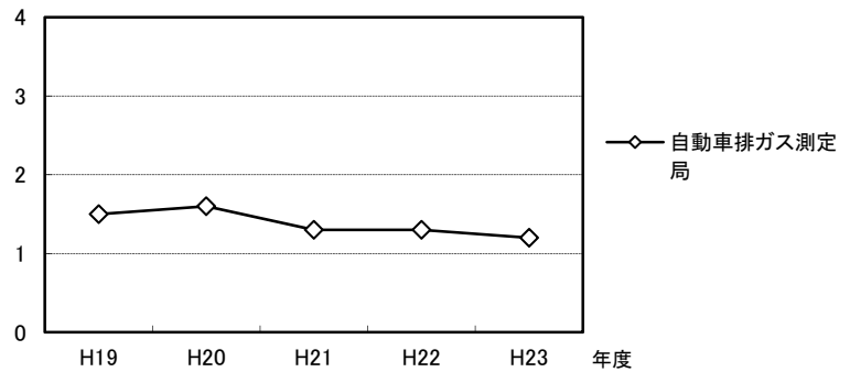
年平均值(ppm) 図表 3-8 ベンゼン濃度の推移
