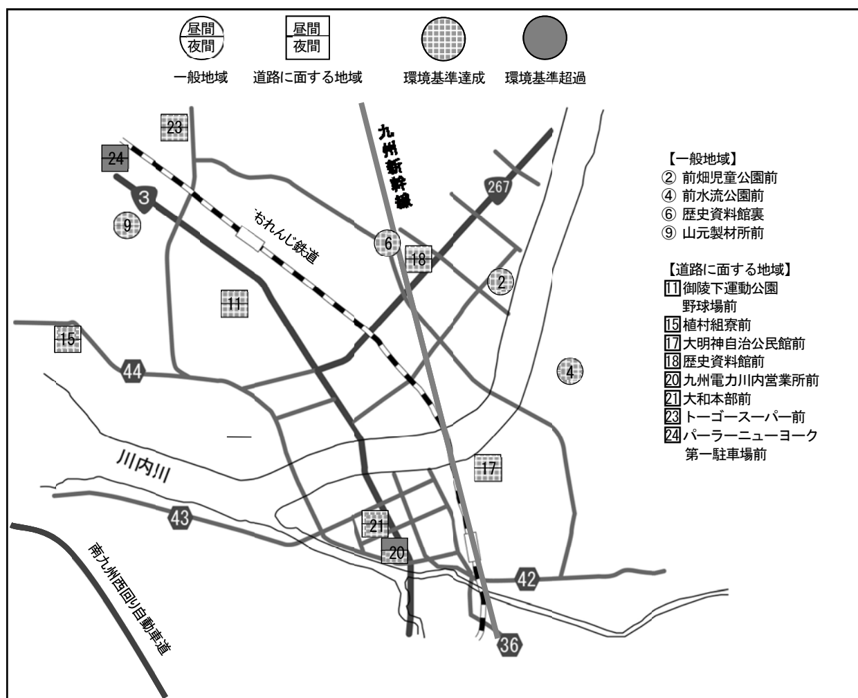
図表 3-10 環境騒音調査の状況（川内地域）
