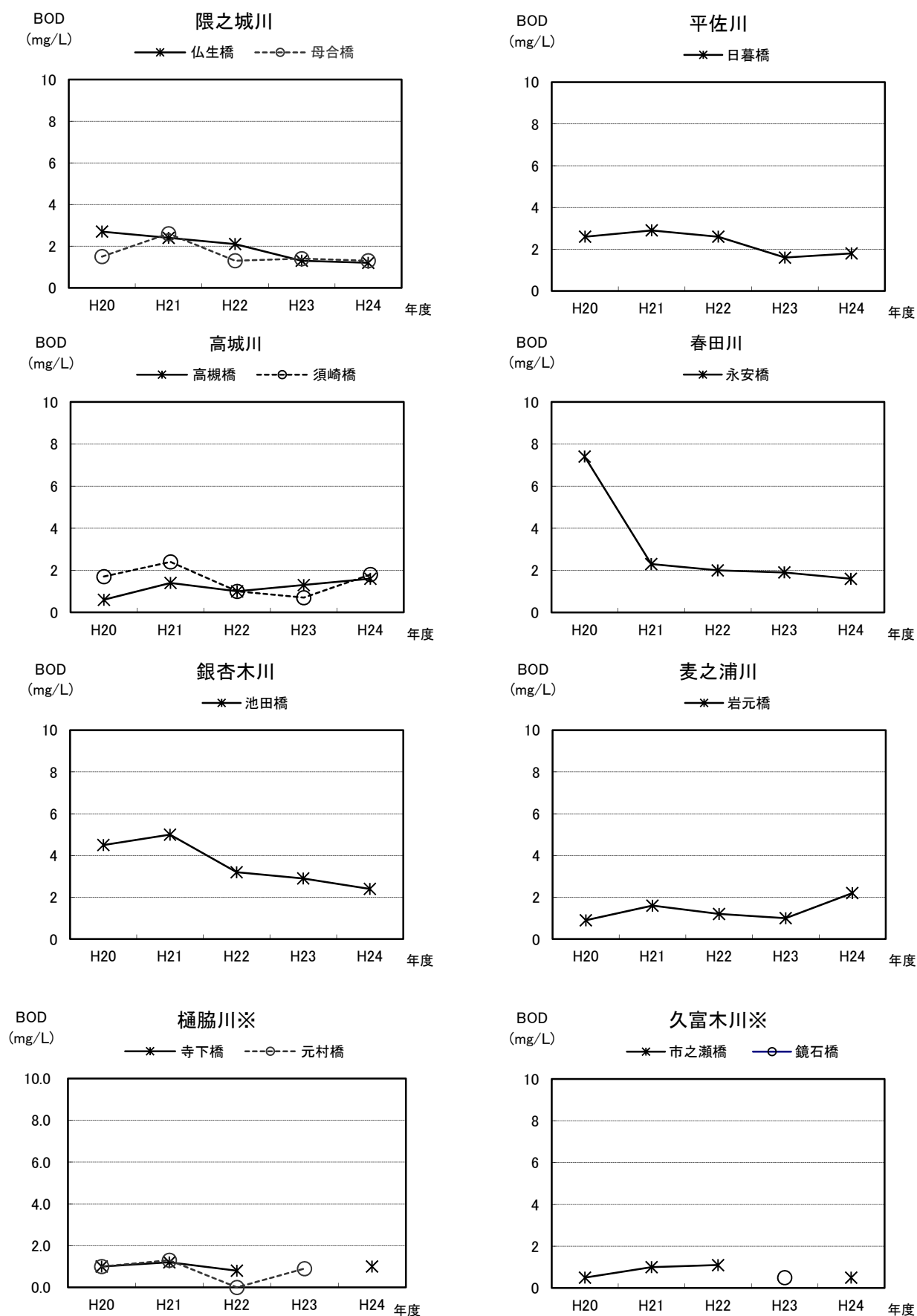
図表 3-14 中小河川の水質の経年変化 〔BOD（生物化学的酸素要求量）の75%値の推移〕
