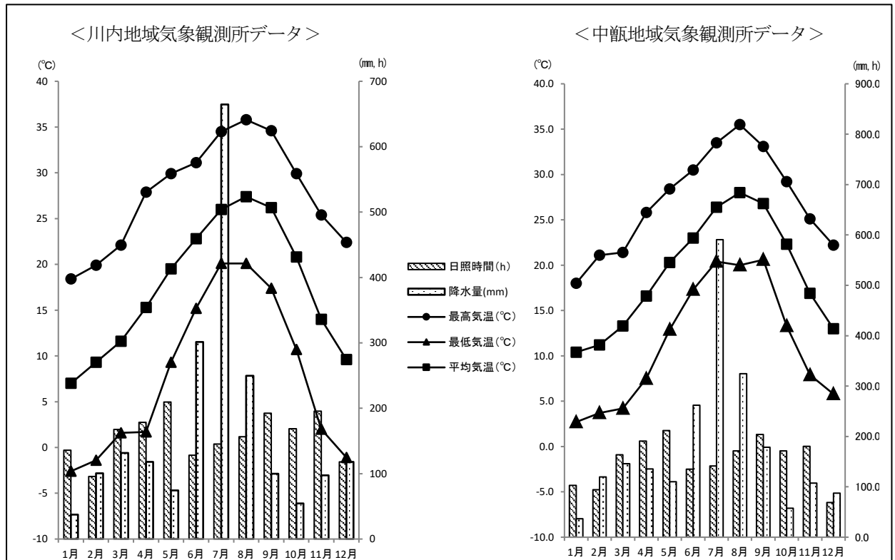
図表 1-1 気温と降水量（令和元年）
