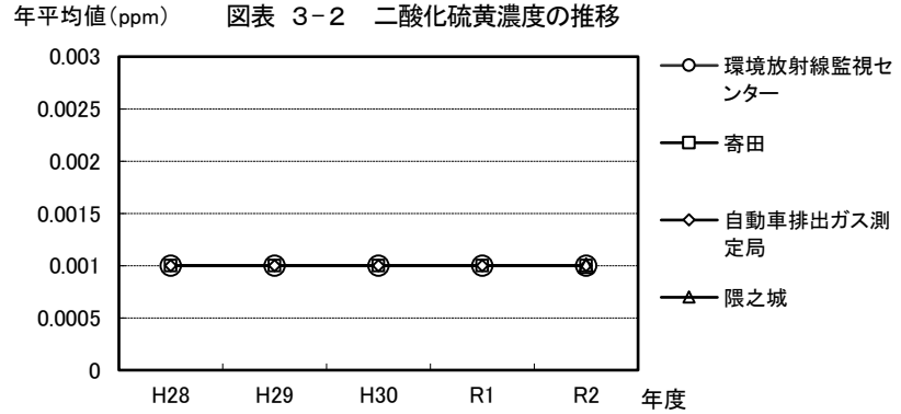
図表 3-2 二酸化硫黄濃度の推移
