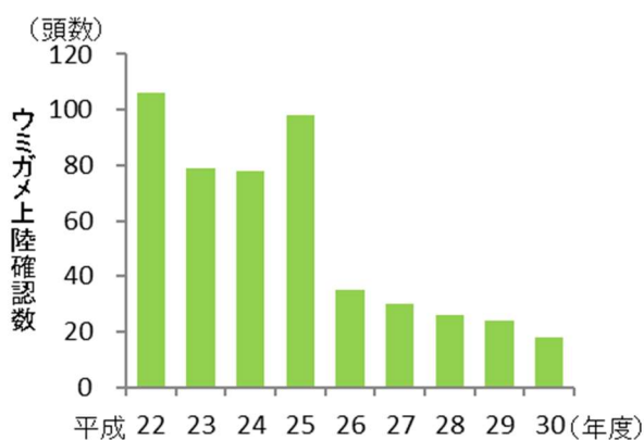
図 3-5-1 ウミガメの上陸確認頭数
