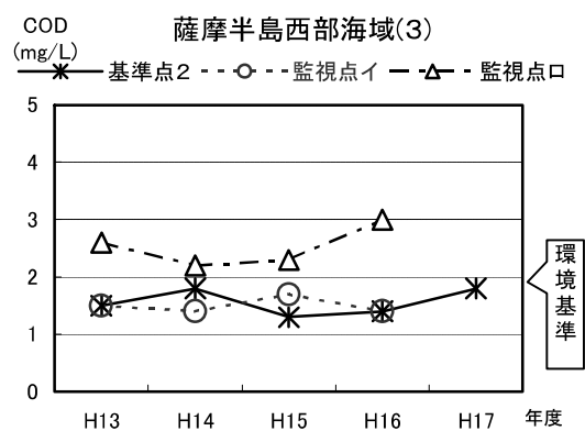
図表 3-13 海域の水質の経年変化
