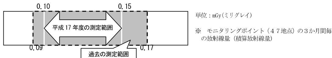
図表 3-18 空間放射線量の状況
