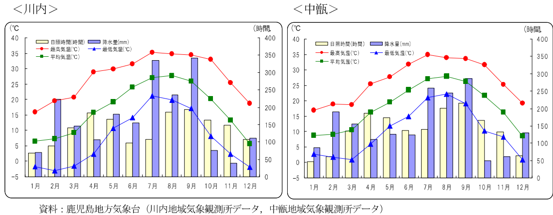
図表 1-1 気温と降水量（平成17年）
