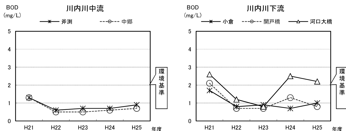
図表3-14 川内川の水質の経年変化
