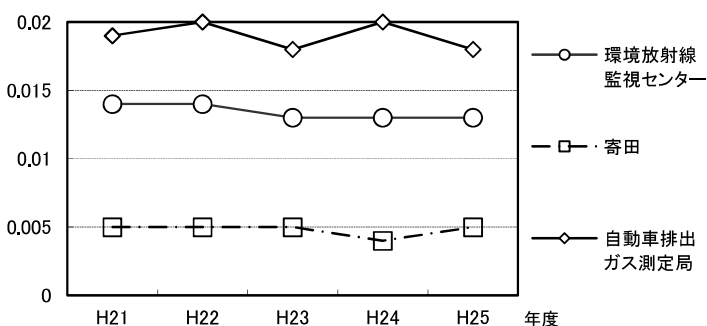
年平均值 (ppm) 図表 3-3 二酸化窒素濃度の推移
