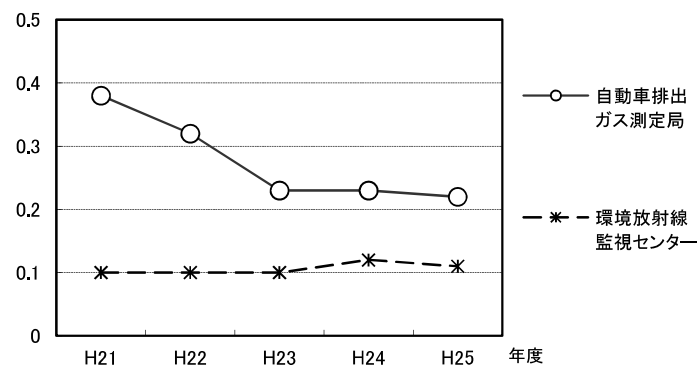
年平均值 (ppmC) 図表 3-7 非メタン炭化水素濃度の推移
