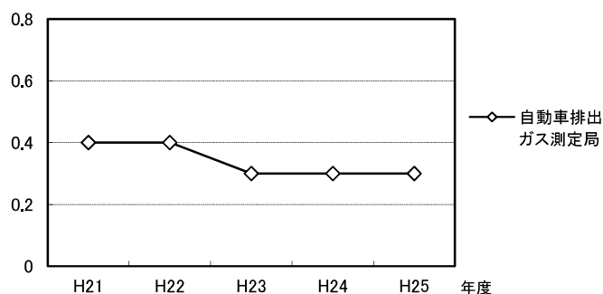
年平均值 (ppm) 図表 3-5 一酸化炭素濃度の推移
