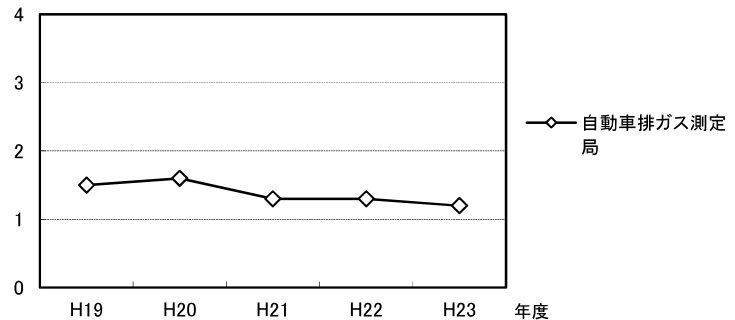
年平均値 (ppm) 図表 3-8 ベンゼン濃度の推移
