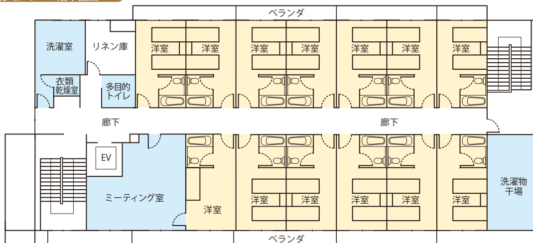
スポーツ交流研修センター3階平面図
