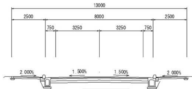
標準断面図
