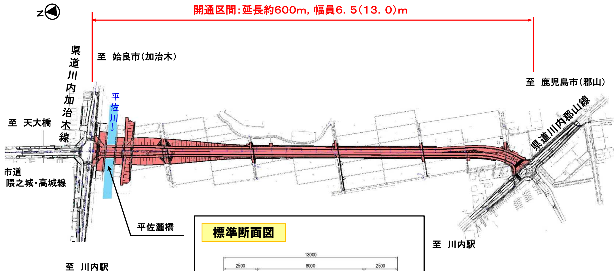
平面図
