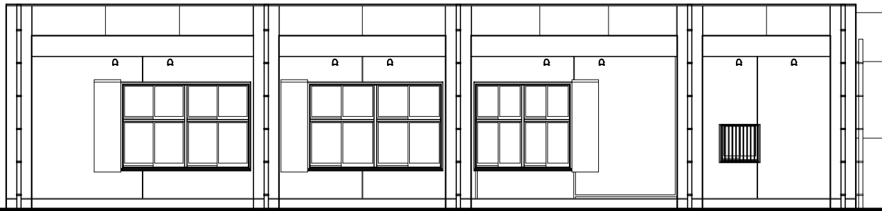
東立面图
