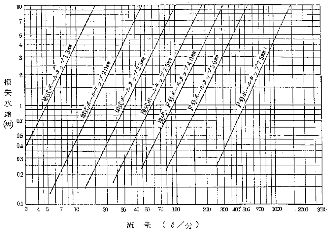
図 4-10 ボールタップの損失水頭
