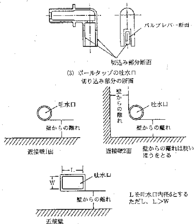
図 4-17 水槽等の場合
