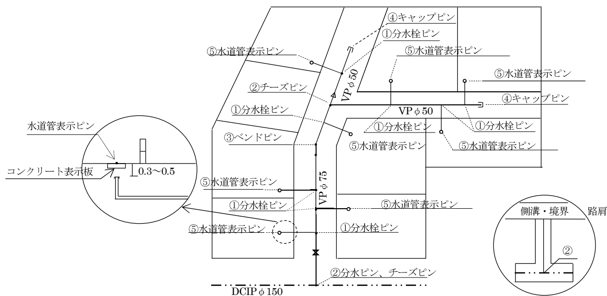
図5-1 水道表示ピン及び水道管表示杭打設要領
