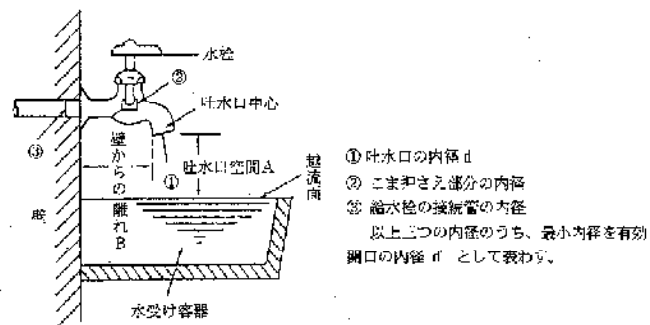
図 4-16 洗面器等の場合
