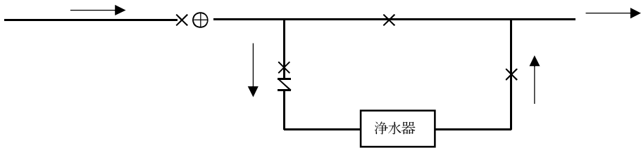
図 4－1 2 バイパス配管の場合 (平面図)
