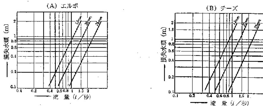
図 4 - 11 継手類による損失水頭
