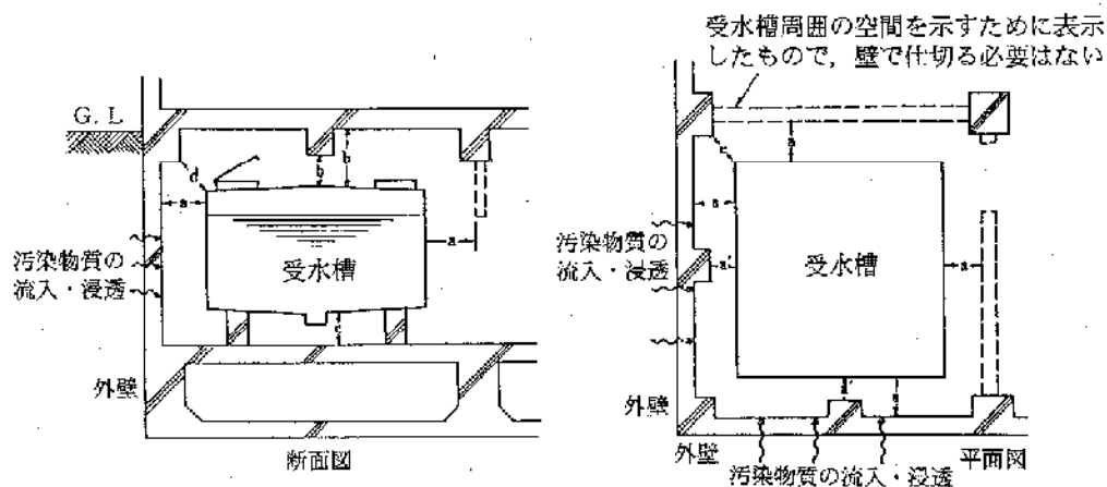
図7-1 受水槽設置位置の一例
