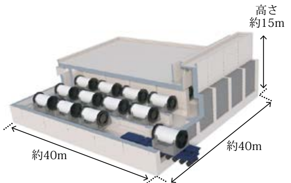
【乾式貯蔵建屋（イメージ）】
