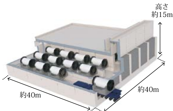
【乾式貯蔵建屋（イメージ）】
